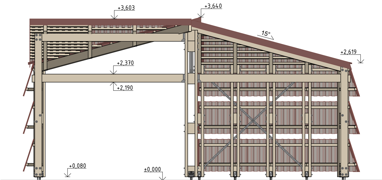
ZÁPADNÍ POHLED
