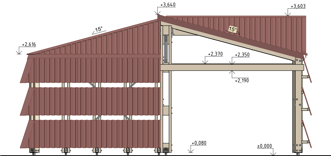
VÝCHODNÍ POHLED
