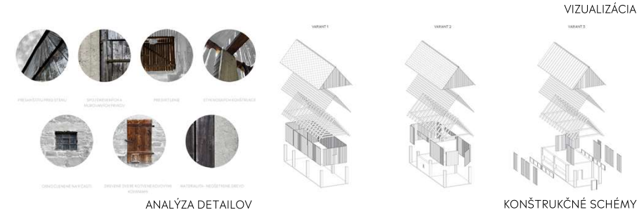
ANALÝZA DETAILOV
