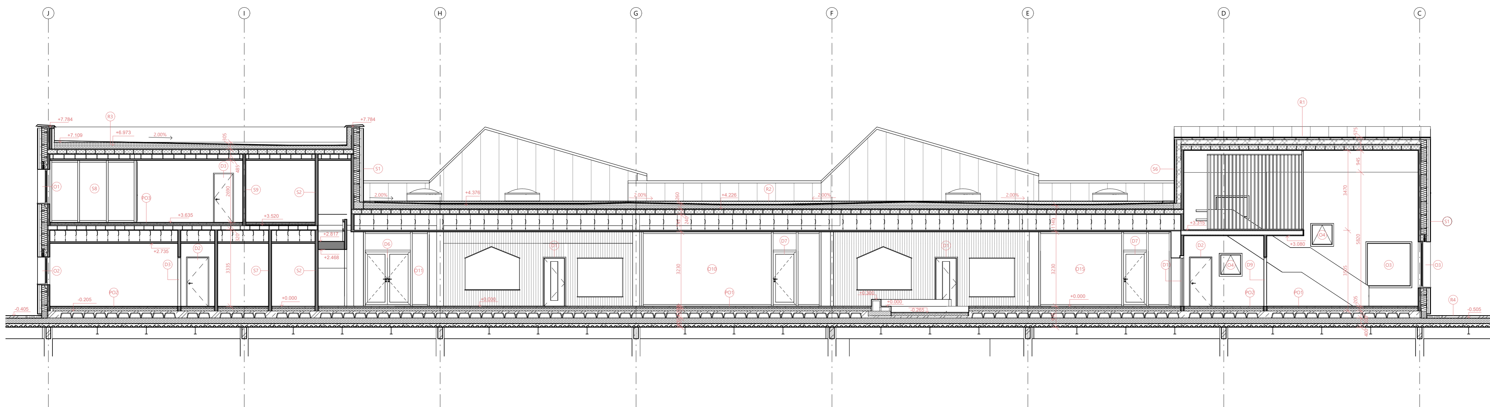
REZ D-D'
