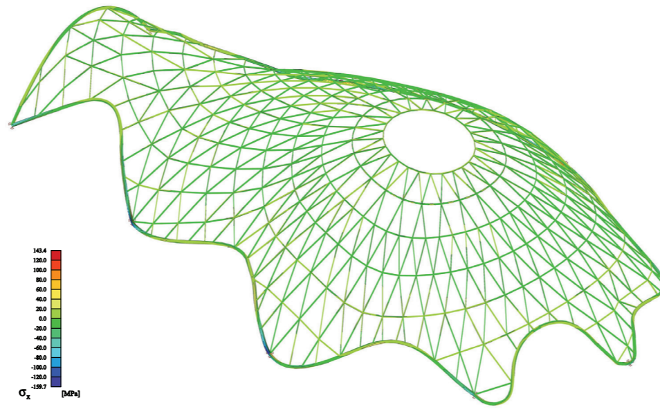
3D NAPĚTÍ
