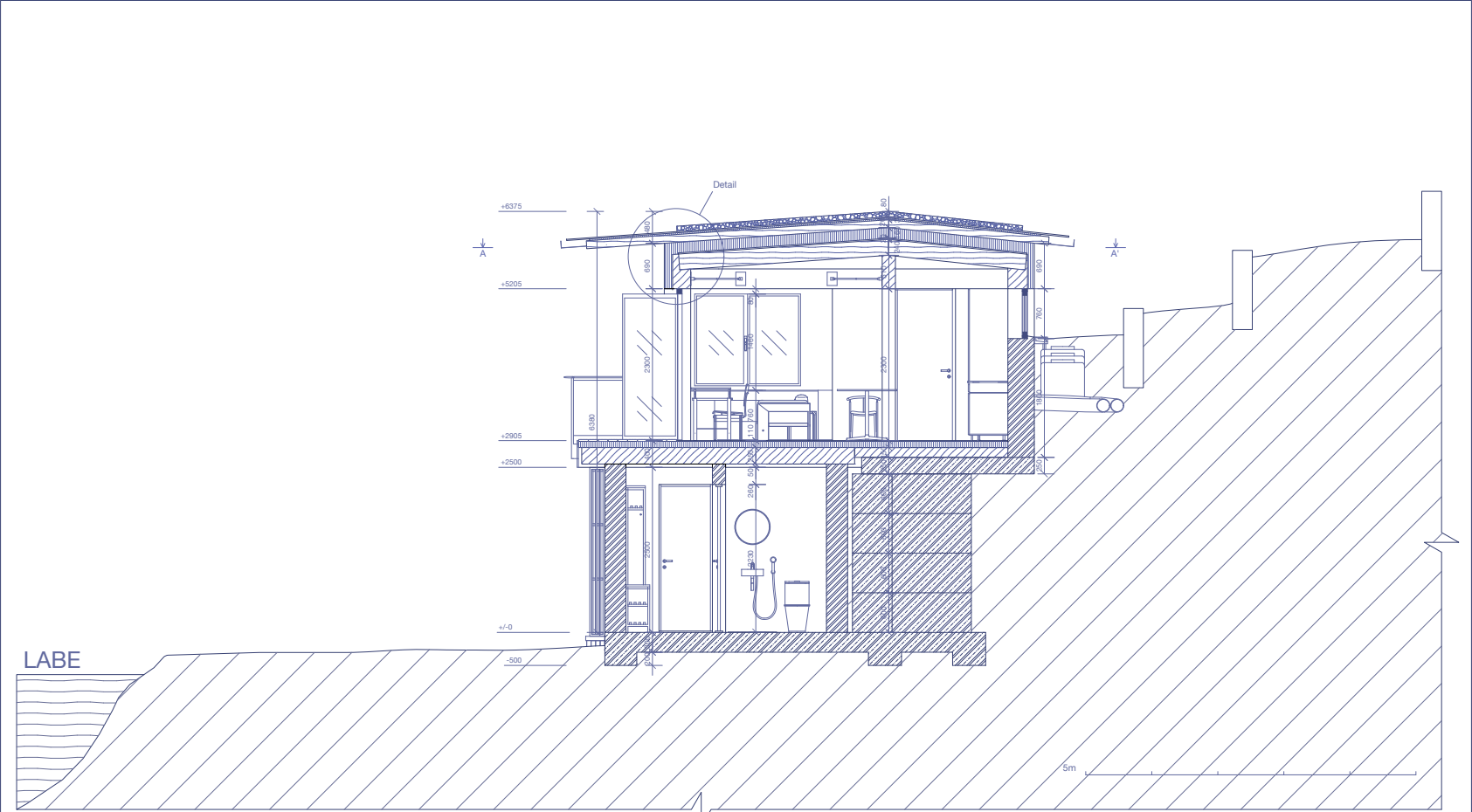
ŘEZ A-A', 1:100
